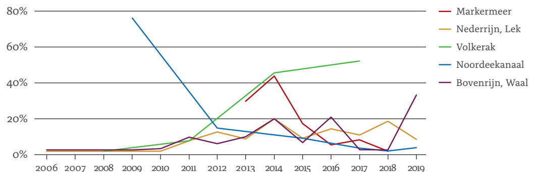
Aandeel zwartbekken per locatie in de periode 2006-2019, gebaseerd op data van boomkorte trekken tijdens de MWTL-monitoring.
